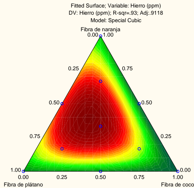
Figura 4: Superficie de respuesta de contorno para la remoción del hierro.
